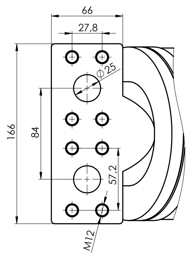
X M 1:2
