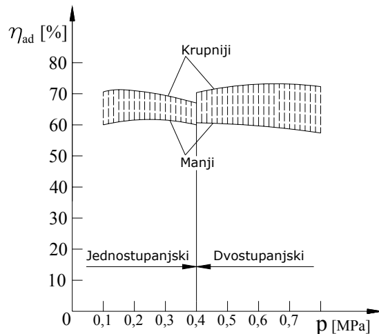
Slika 20. Zavisnost opće adijabatske iskoristivosti \eta_{ad} o povećanju tlaka za jednostupanjski i dvostupanjski zračni kompresor
