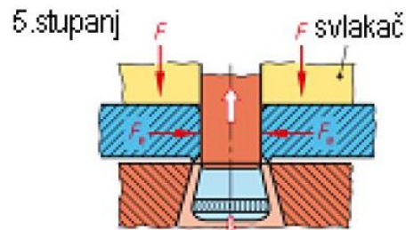
Slika 8. 5. stupanj rezanja na štancama [2]
