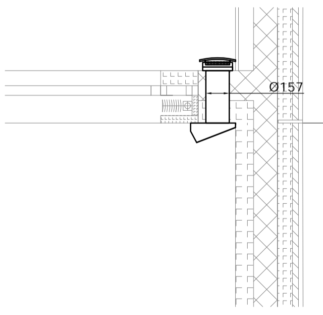
Detalji 1 - ugradnja ventilacijskog ure aja iznad prozora M1: 25
