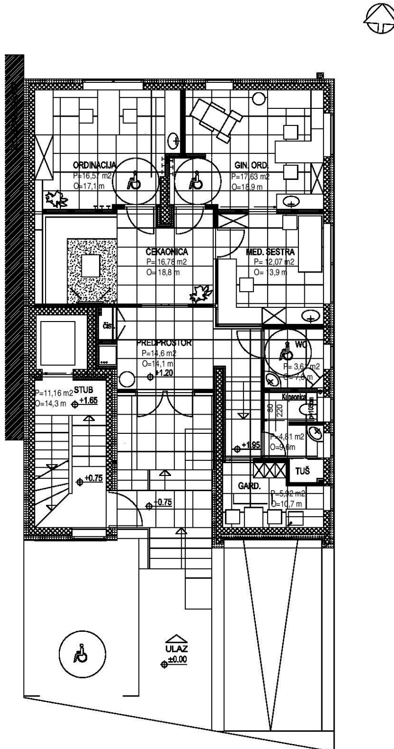
Slika 10. Tloert prizemlja
