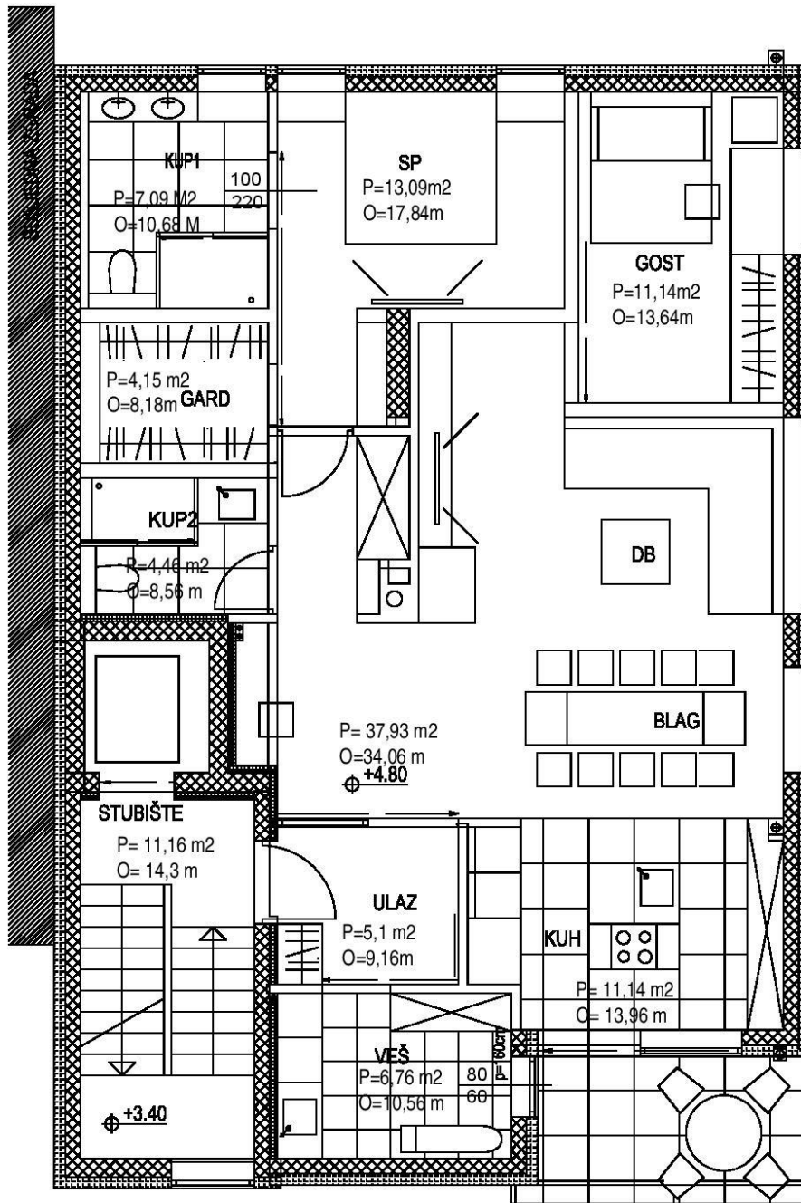
Slika 11. Tloert 1. kata
