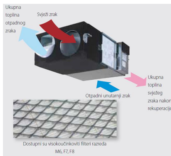
Slika 30. Ventilacijska jedinica VAM-800 FC [13]
