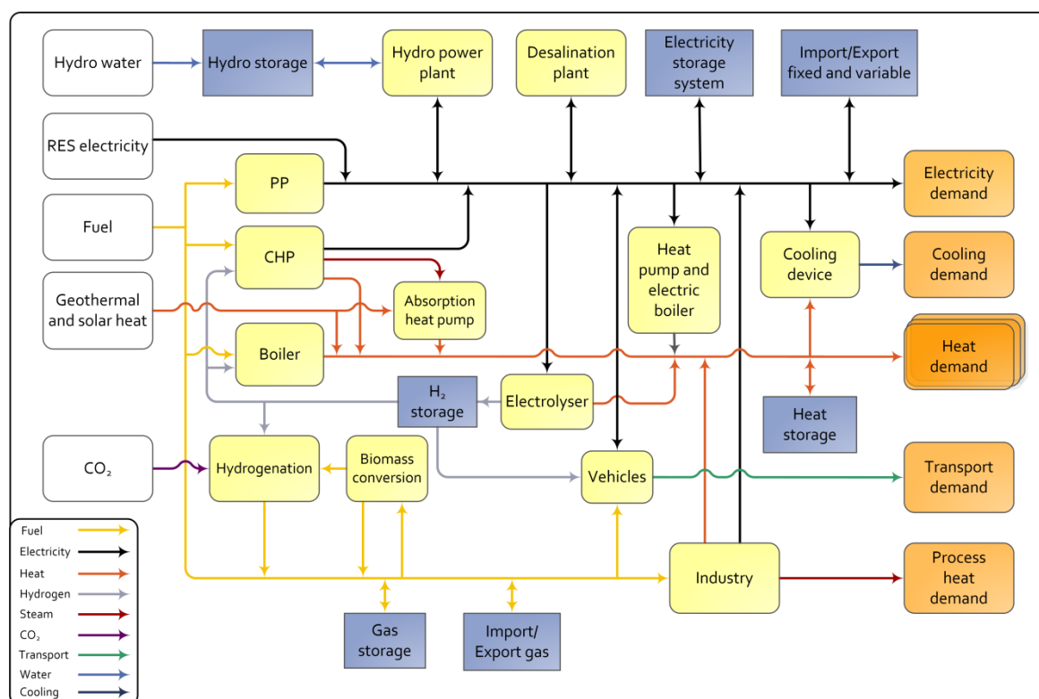
Slika 21. EnergyPLAN model [32]
