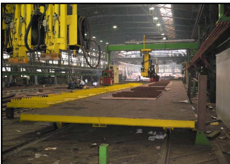
Slika 1. Radna platforma automatizirane linije
