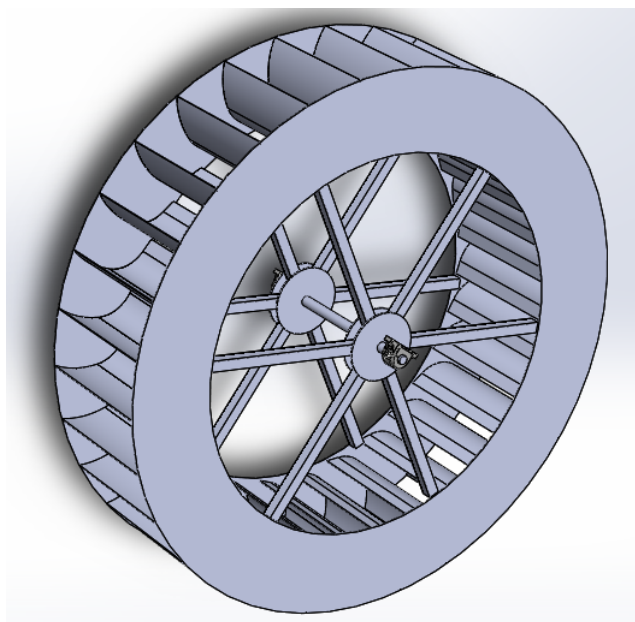
Slika 4.1: Izometrijski prikaz geometrije kola [6]
