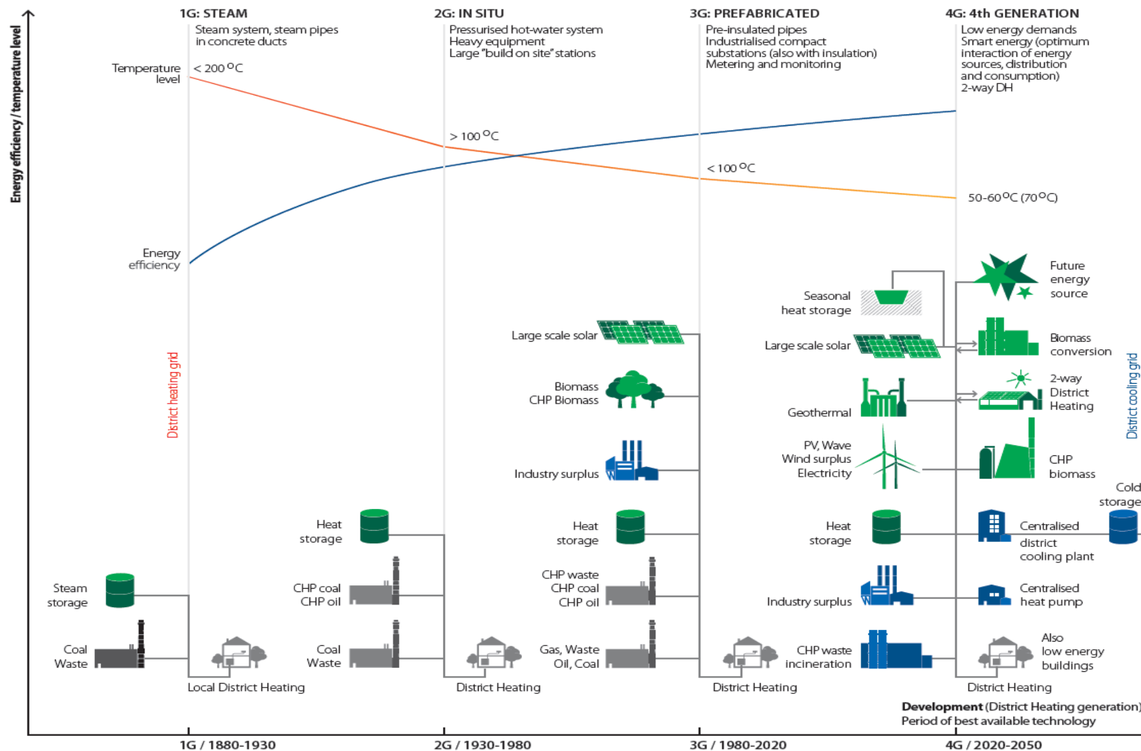
Slika 2 Razvoj centraliziranih toplinskih sustava [22]
