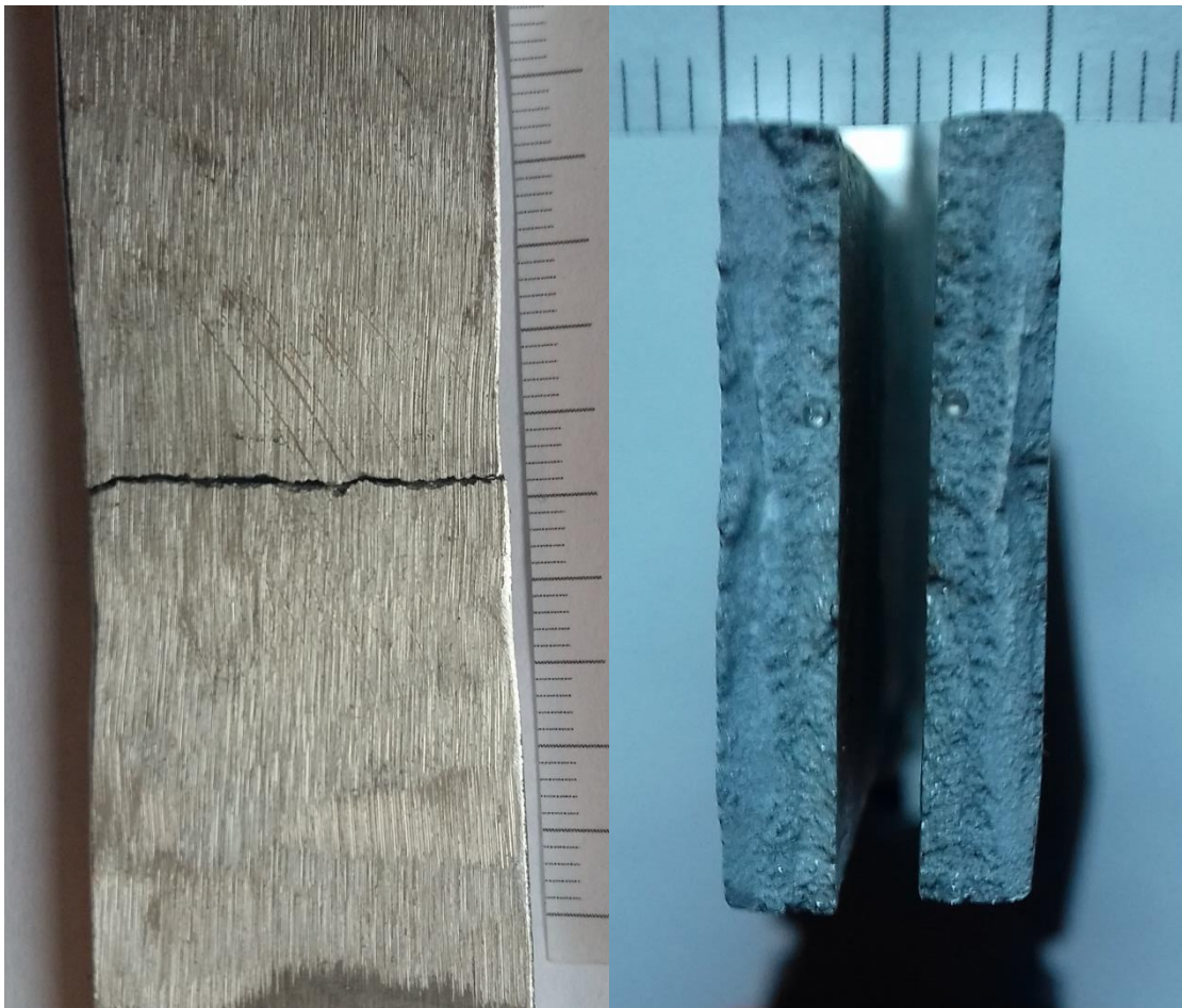
Slika 62. Epruveta 3-5
