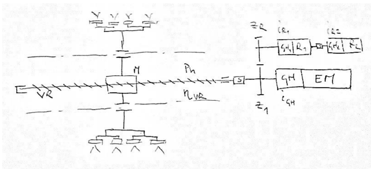
Slika 6.1 Shema pogona translacije
