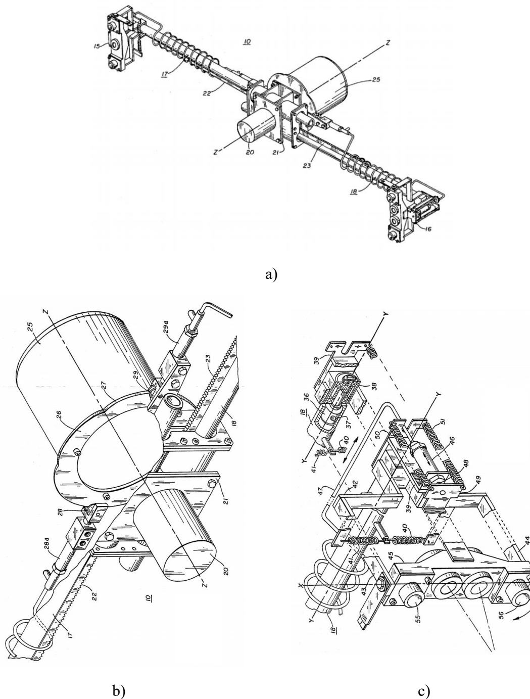
Slika 2.14 US4368644, 1983. godina a) modul za ispitivanje b) bregasti prsten c) hidraulički aktuator
