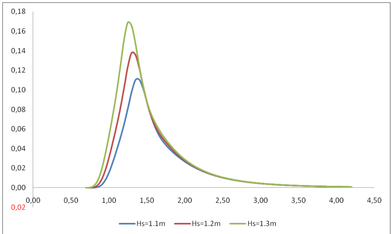
Slika 11. Tabainov spektar za zadane značajne valne visine
