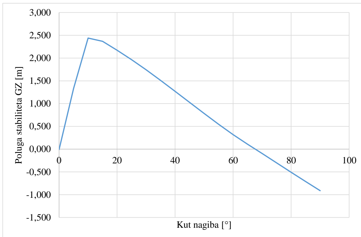
Slika 34. Poluga stabiliteta
