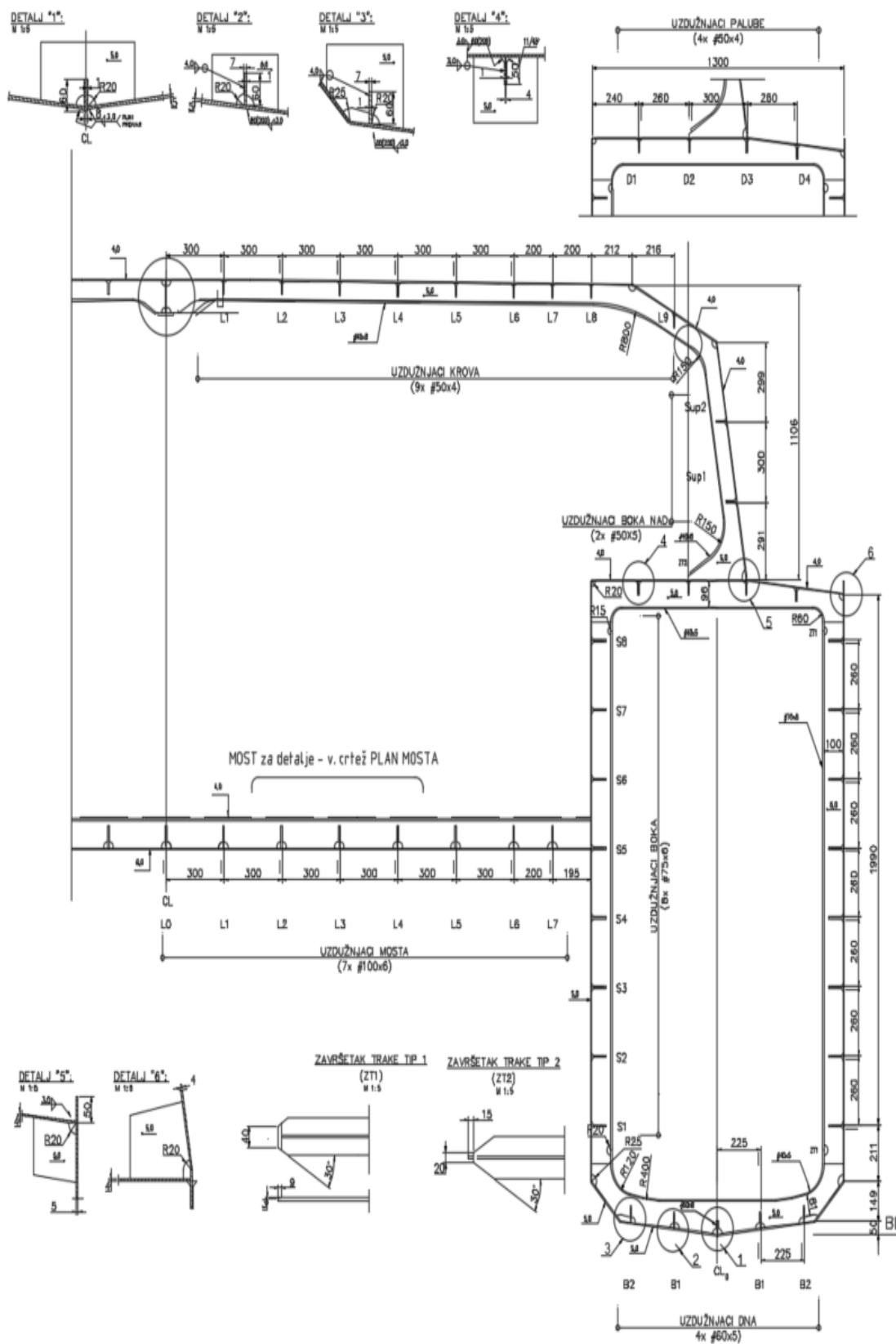
Slika 33. Glavno rebro
