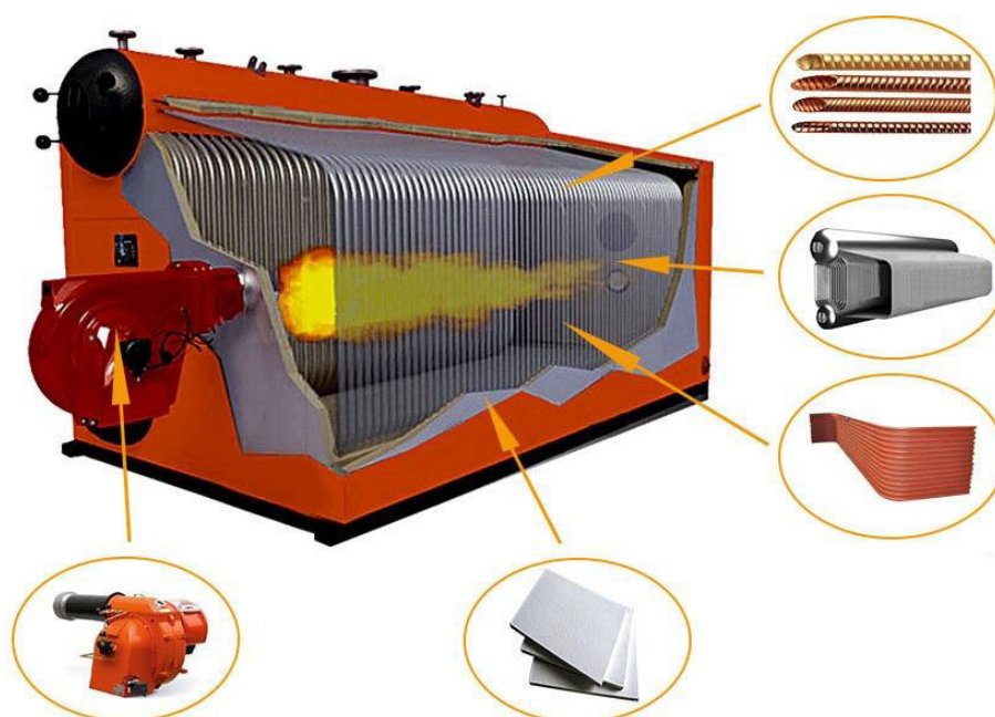
Slika 1. Vodocijevni kotao [1]
