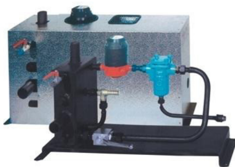
Slika 10. Modul optoka ulja OCM
