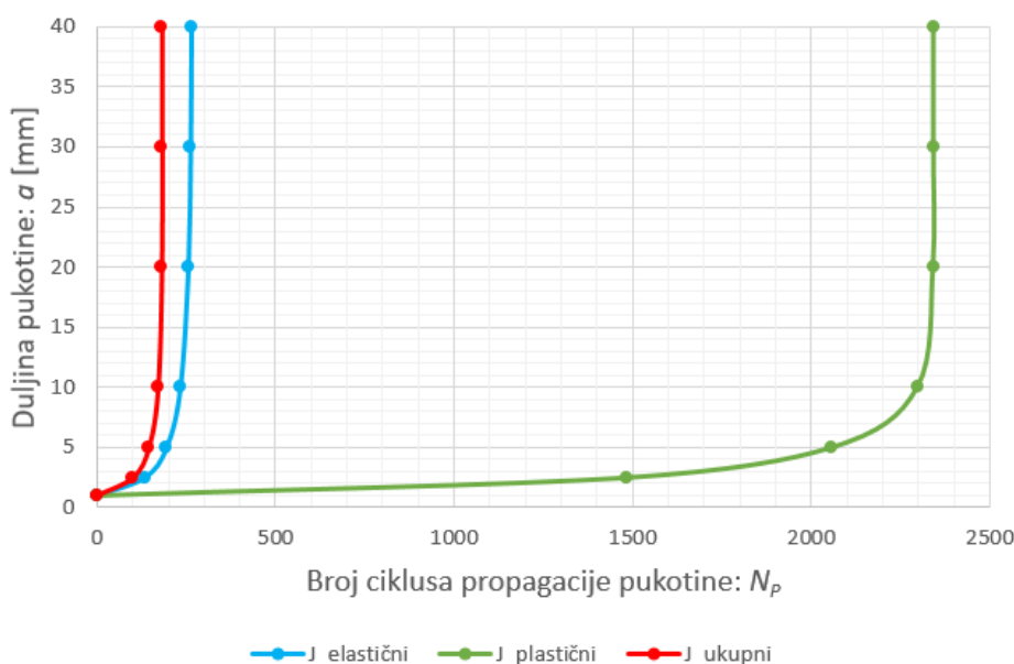
Slika 64. Usporedba broja ciklusa do loma za elastični, plastični i ukupni J -integral
