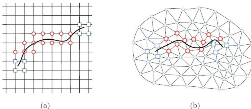
Slika 16. Selekcija "obogaćenih" čvorova 2D analize s pukotinom za jednoliku mrežu (a) i nejednoliku mrežu (b) [4]
