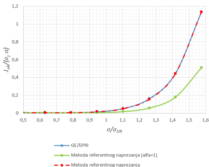
Slika 53. Usporedba GE/EPRI metode i MRN metode s obzirom na ukupni J -integral i omjer opterećenja ( a = 10 \text{ mm} , t = 10 \text{ mm} )
