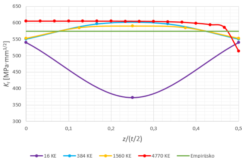
Slika 38. Konvergencija koeficijenta intenzivnosti naprezanja po debljini ploče t = 10 mm, duljine pukotine 2a = 20 mm i opterećene \sigma = 100 MPa
