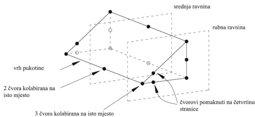
Slika 14. Sažimanje prizmatičnog konačnog elementa za 3D analizu [7]
