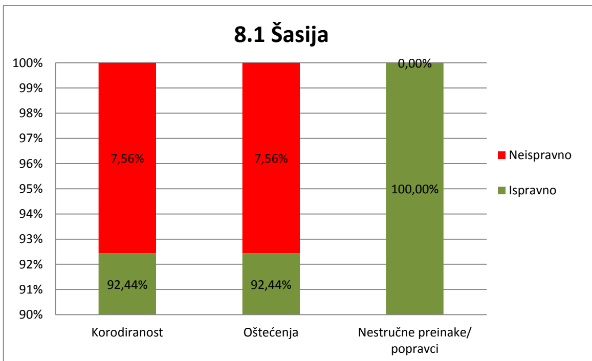
Slika 5.3. Dijagram neispravnosti pojedinih podsklopora za šasiju
