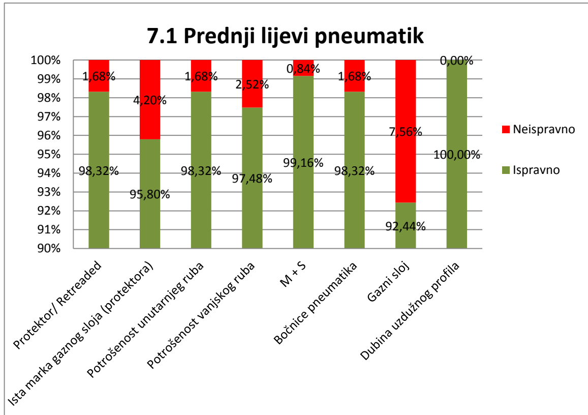
Slika 5.2. Dijagram neispravnosti pojedinih podsklopora za prednji lijevi pneumatik
