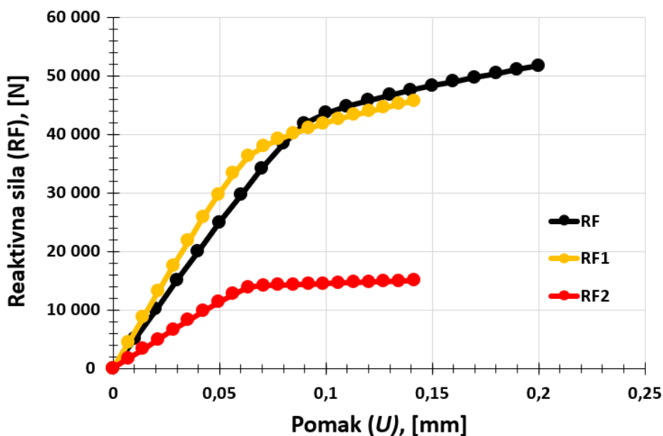
Slika 6.6. Dijagram sila-pomaka za kombinirano opterećenje (45°)
