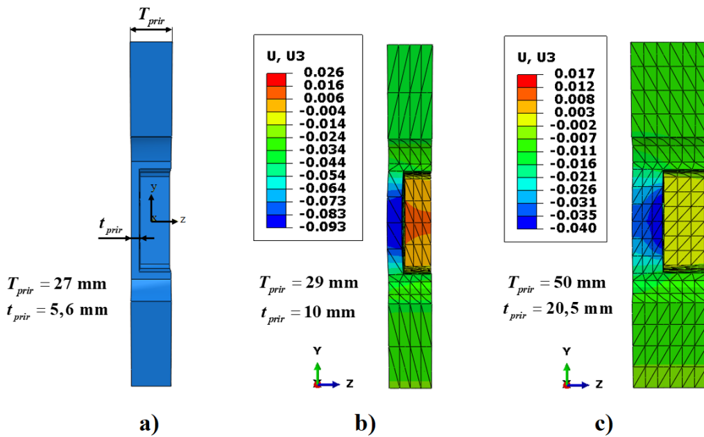
Slika 7.6. Utjecaj pomaka U_3 ovisno o debljini prirubnice pri deformaciji \approx 20\% : a) početna geometrija, b) T_{prir} = 29 mm, c) T_{prir} = 50 mm
