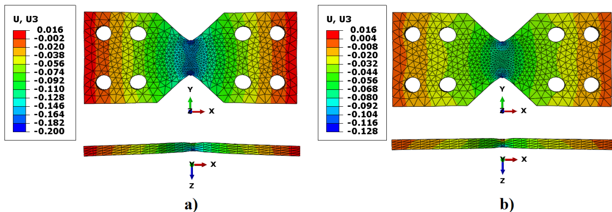
Slika 7.7. Savijanje leptirastog uzorka pri deformaciji \approx 20\% ovisno o debljini prirubnice: a) T_{prir} = 29 mm, b) T_{prir} = 50 mm
