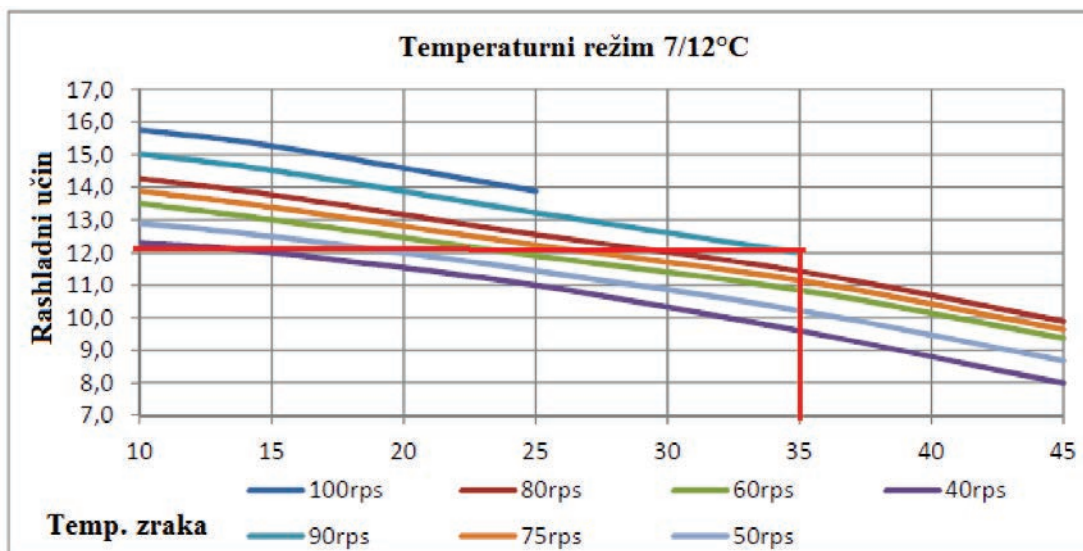
Slika 17: Rashladni učin dizalice topline u ovisnosti o temperaturnom režimu [7]
