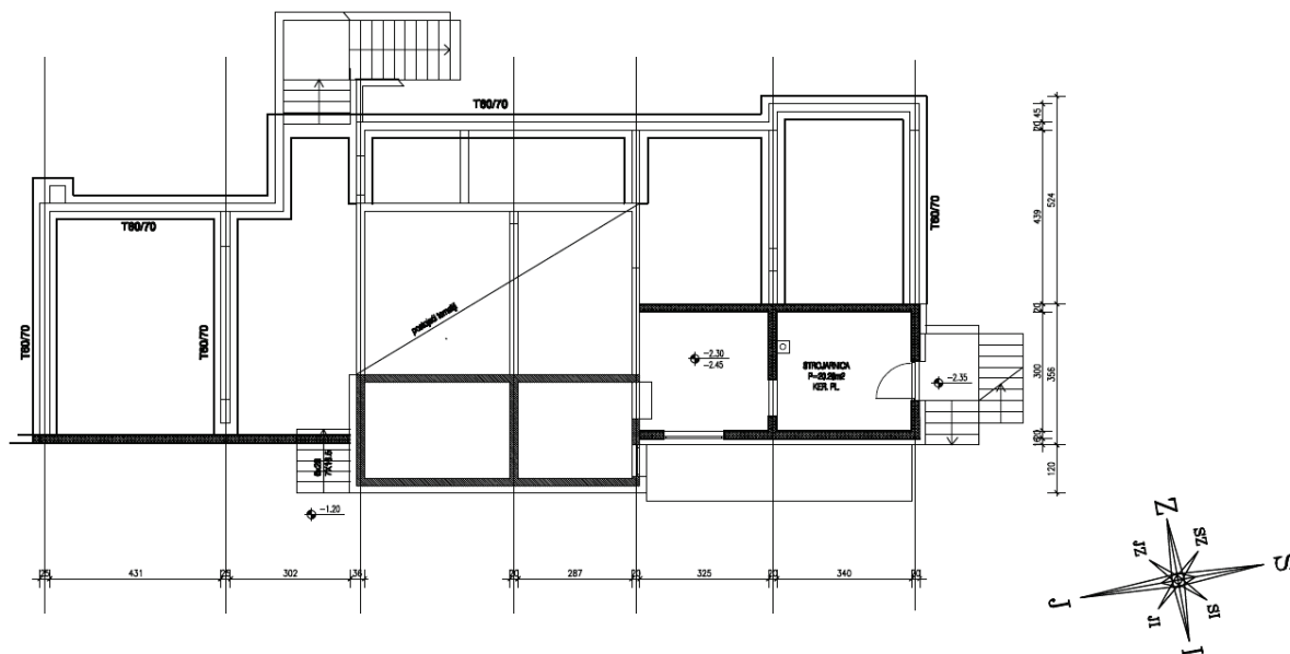
Slika 11: Tlocrt podruma
