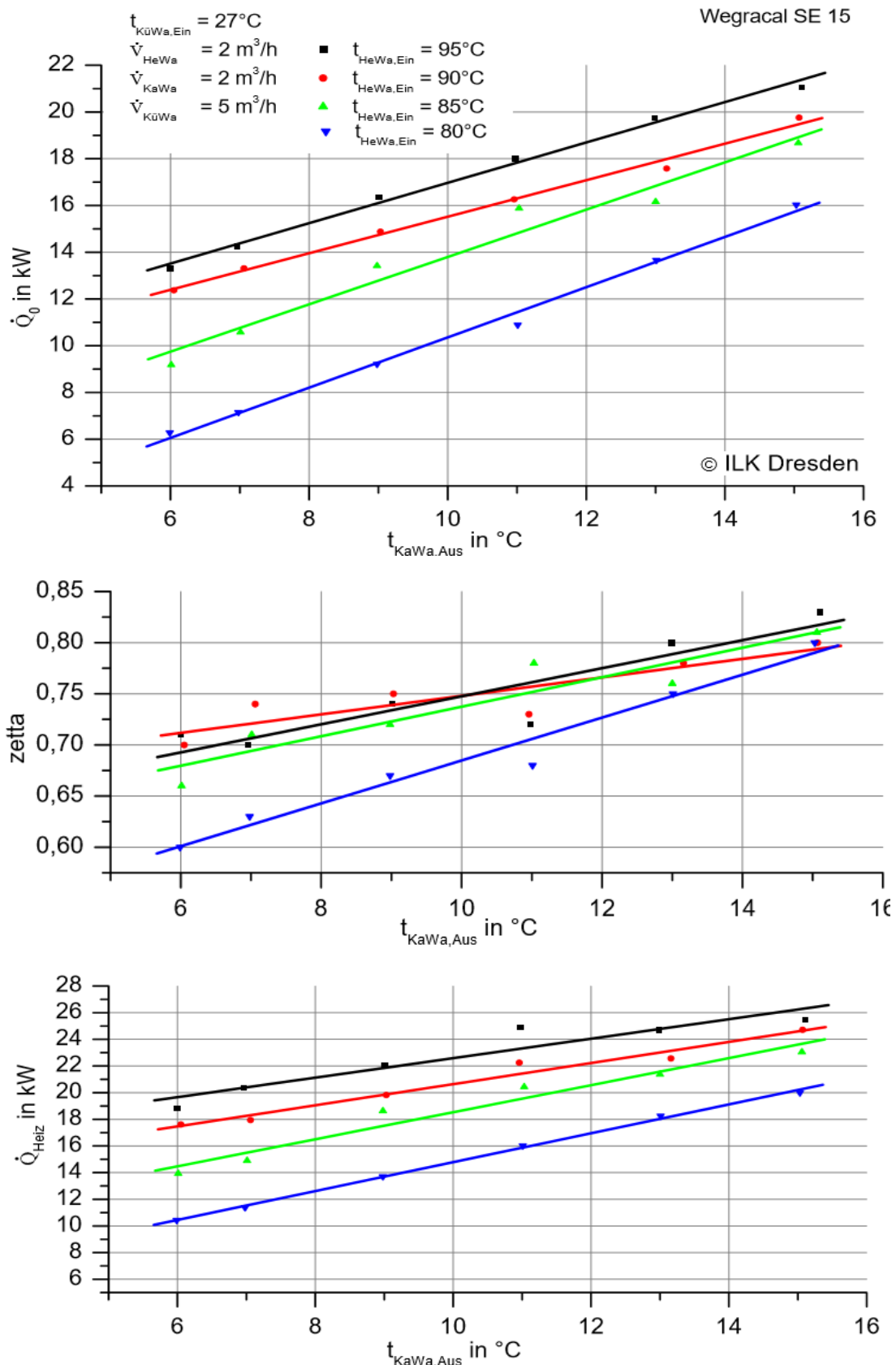
Slika 2.14. Potrebna ogrjevna snaga, učinkovitost i rashladna snaga Wegracal 15 u ovisnosti o izlaznoj temperaturi hladne vode i temperaturi ogrjevne vode [9]
