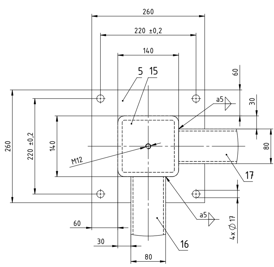
G (1 : 5)
