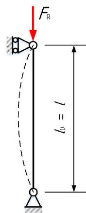
Slika 36 Proračunski model izvijanja
