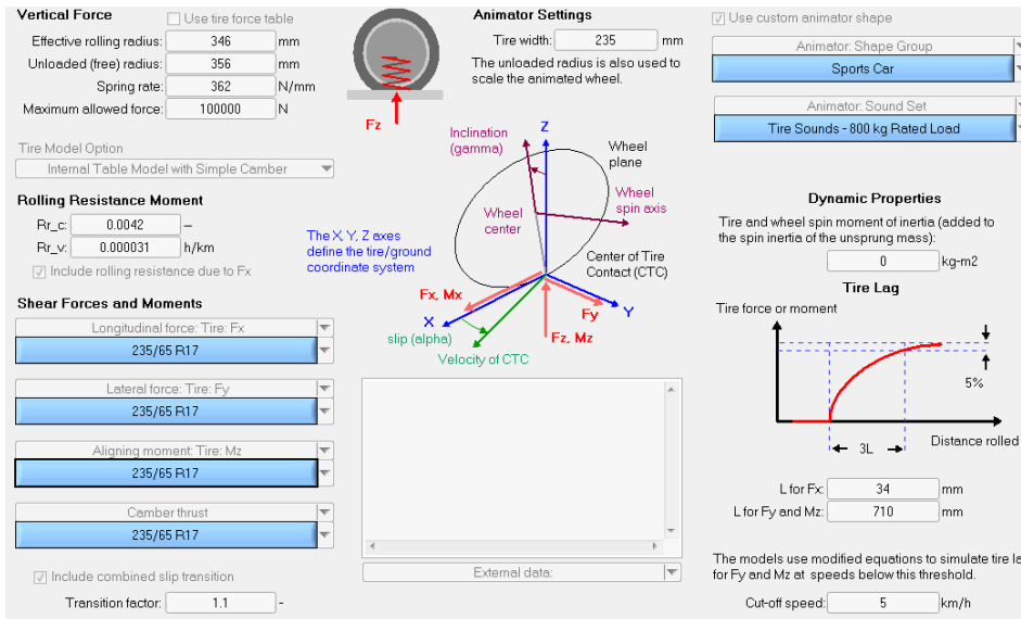
Slika 44. Karakteristike pneumatika
