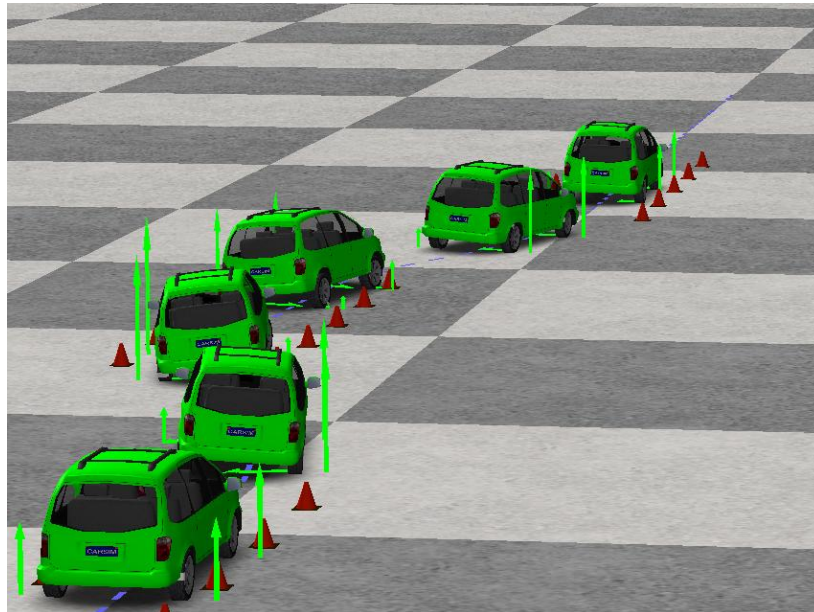
Slika 8. Simulacija dvostruke izmjene pravca u CarSim programskom paketu
