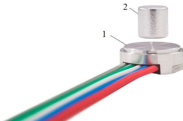
Slika 68. Rotacijski magnetski enkoder RLS RM08 [49]
