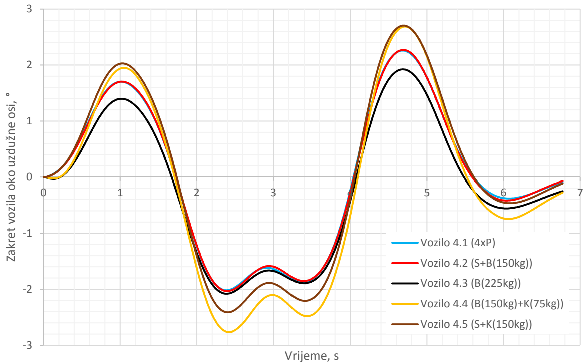
Slika 56. Utjecaj razmještaja tereta/putnika u vozilu kut zakreta vozila oko uzdužne osi
