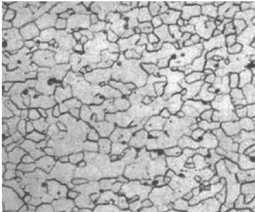
Slika 2. Mikrostruktura feritnog čelika [5]
