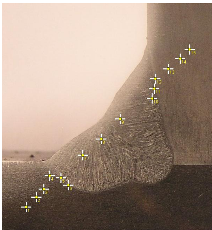
Slika 51. Pozicije mjerenja tvrdoće na uzorku 1
