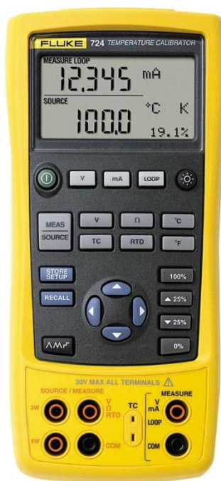
Slika 16. Termometar Fluke 724
