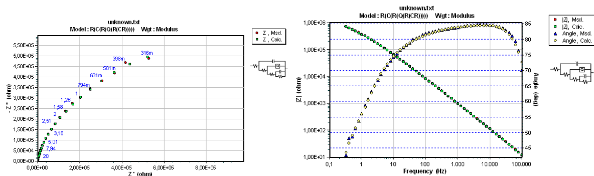
Slika 49. Bodeov i Nyquistov dijagram za uzorak 500
