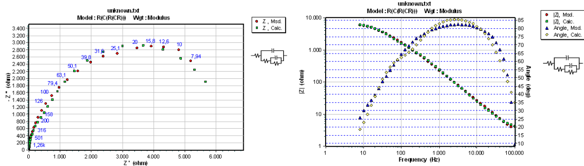
Slika 47. Bodeov i Nyquistov dijagram za uzorak 100
