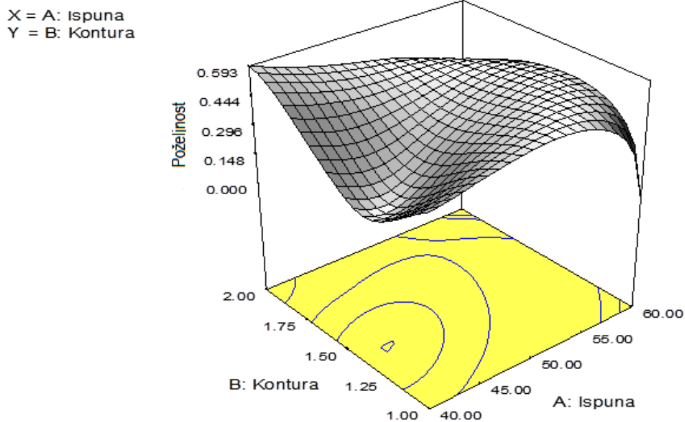
Slika 9.5. Graf ovisnosti funkcije poželjnosti (kompleksna funkcija) o ispuni i konturi pri kompleksnom optimiranju
