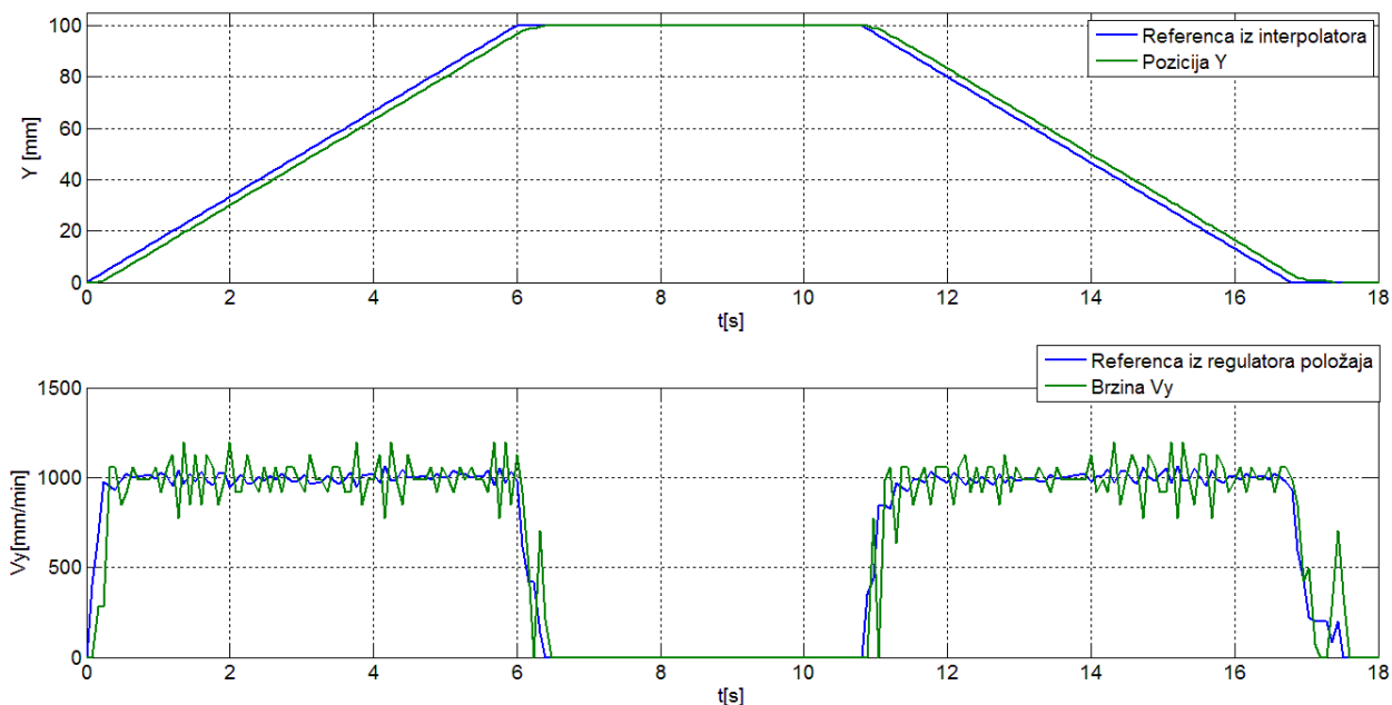
Slika 33. Odziv Y osi za vrijednosti: K_{PY}=400 , K_{RY}=0.001 , K_{IY}=0.04 , F=1000
