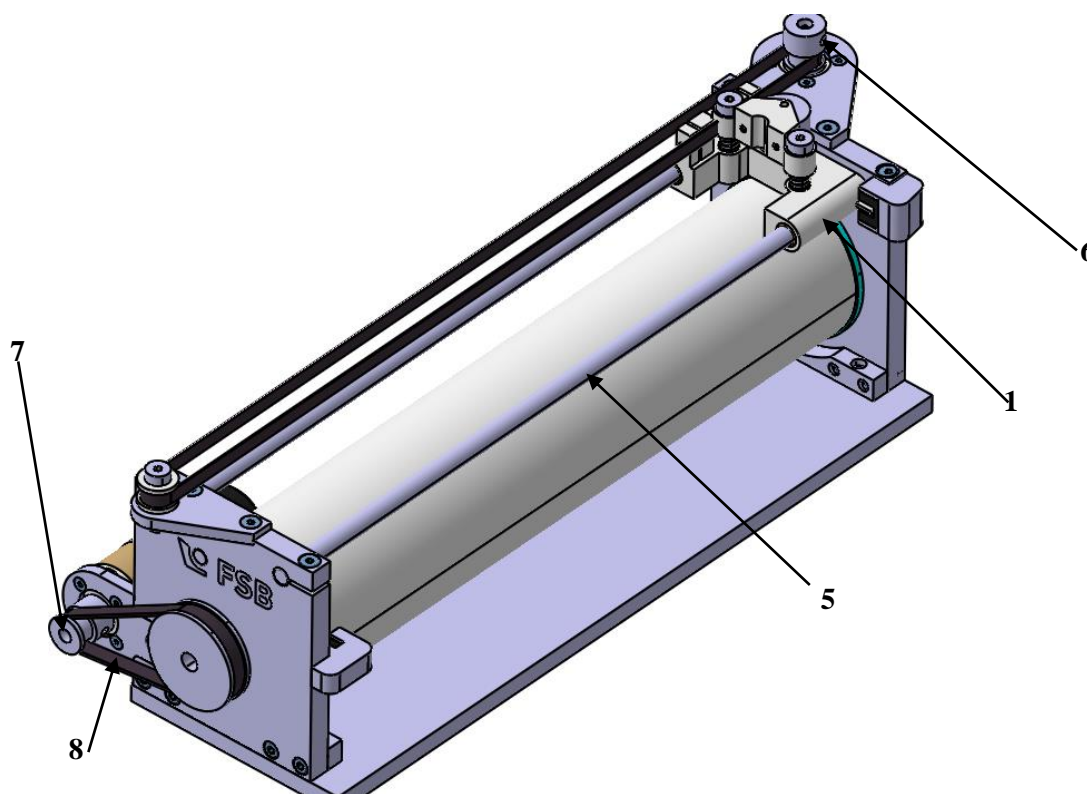
Slika 6. CAD model 1
