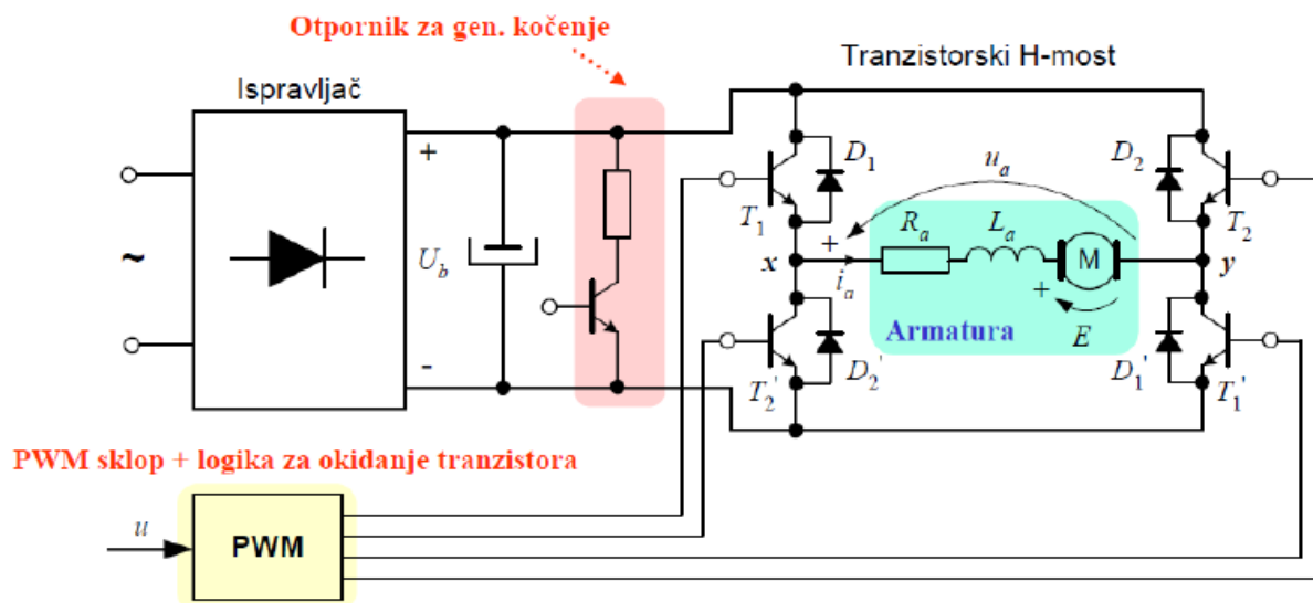
Slika 34. Shema H-mosta [14]
