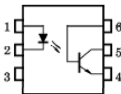
Slika 49. Shema 6 pinskog optokaplera [26]
