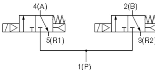
Slika 15. Simbol razvodnika 3/2 [10]
