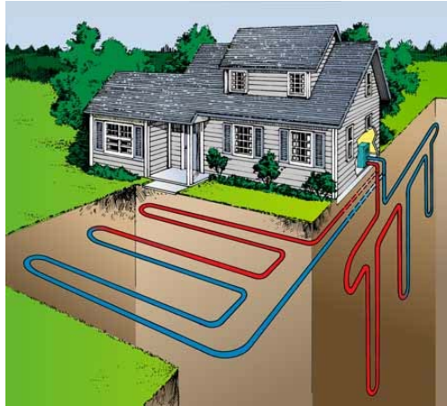
Slika 6. Primjer podzemnih toplinskih kolektora i sonde
