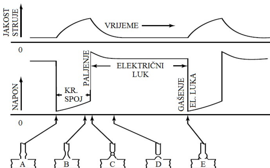
Slika 3. Dijagramski prikaz ovisnosti struje i napona tijekom kratkoga spoja [7]
