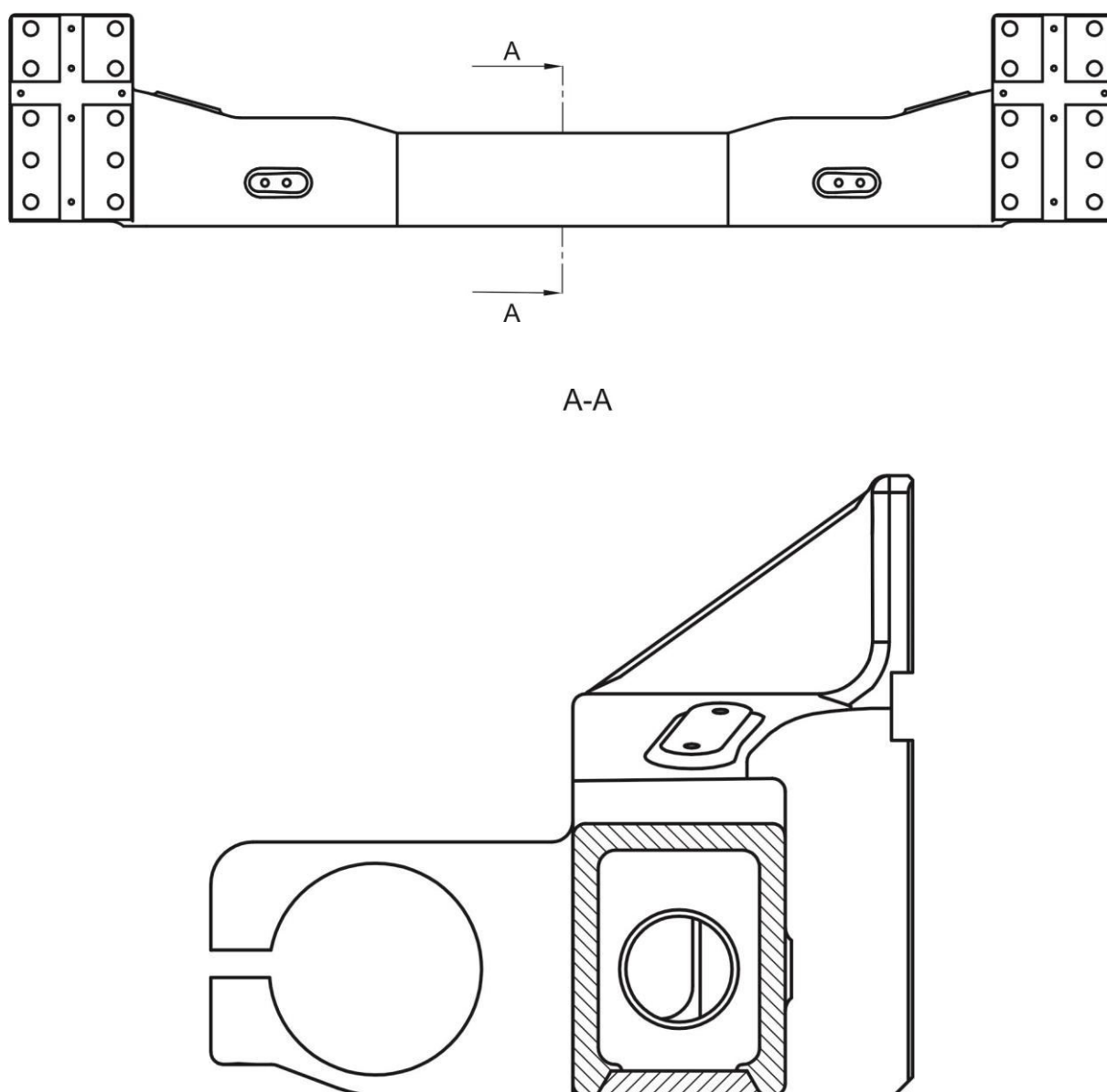
Slika 16. Presjek A-A
