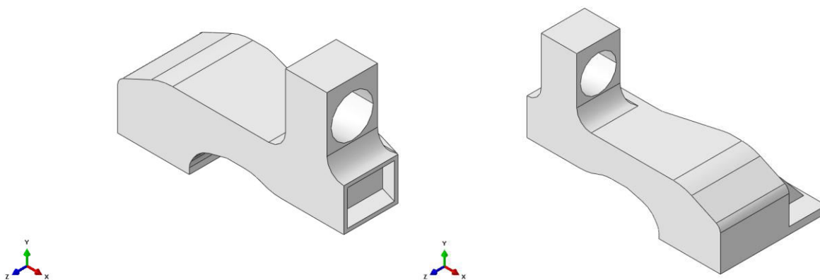
Slika 31. Lijevo (lijevo) i desno (desno) kraj vodilice
