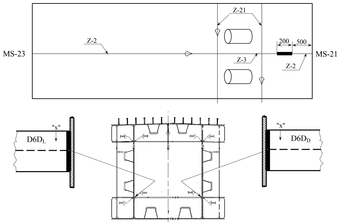
Slika 18: Položaji indikacija (zatomnjeno) na gornjoj pojasnici (gore) i na zavaru Z41 dijafragma D6D (dolje) [25]
