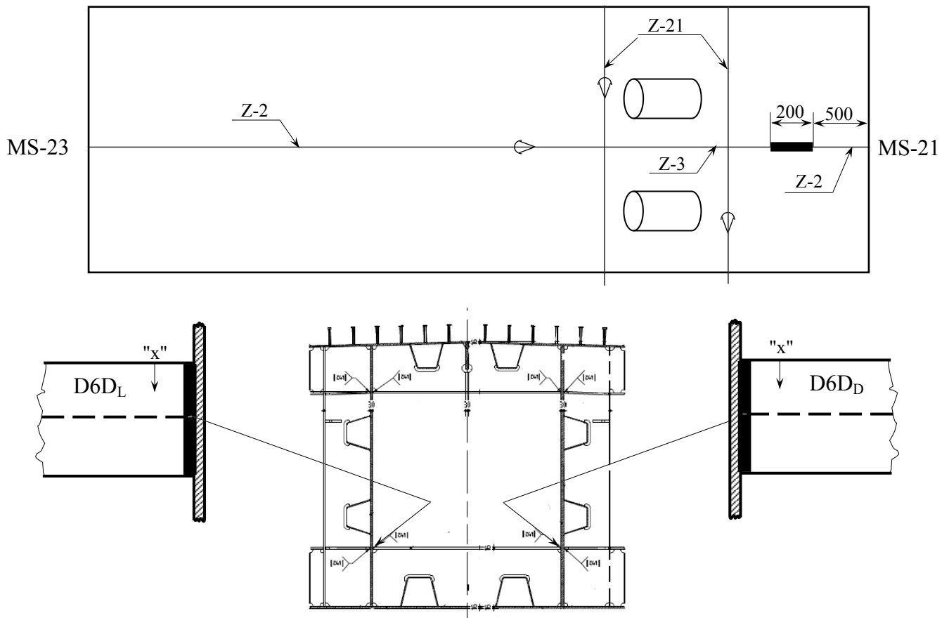
Slika 18: Položaji indikacija (zatomnjeno) na gornjoj pojasnici (gore) i na zavaru Z41 dijafagma D6D (dolje) [25]
