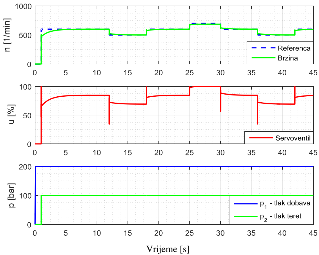
Slika 37 Simulacijski rezultati - rotacija
