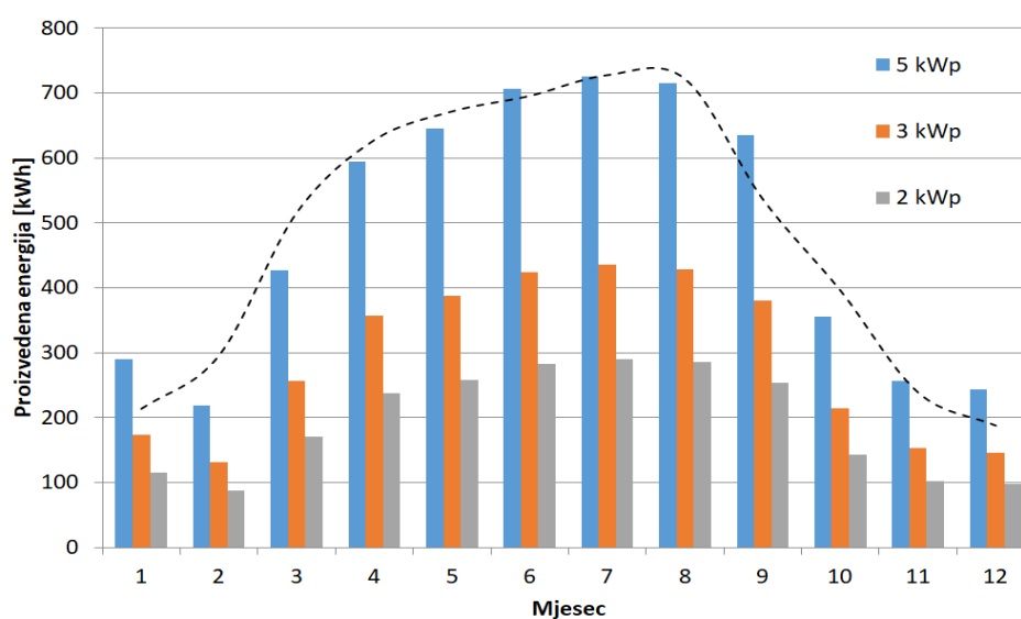
Slika 10. Ukupna mjesečna proizvedena energija u 2016. godini
