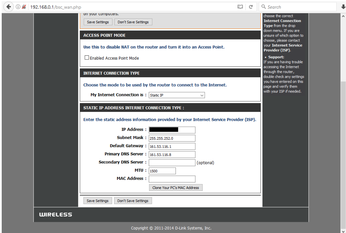
Slika 18: Definiiranje statičke IP adrese routera
