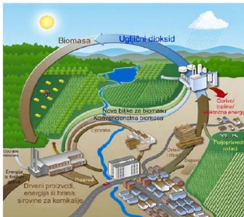
Slika 1. Ciklus biomase [1]
