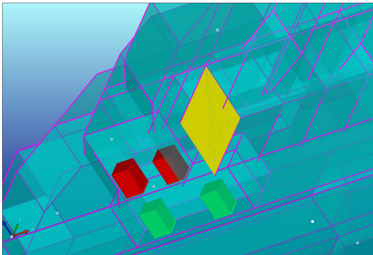
Slika 32. Promjena debljine stijenke oplata prostorije
