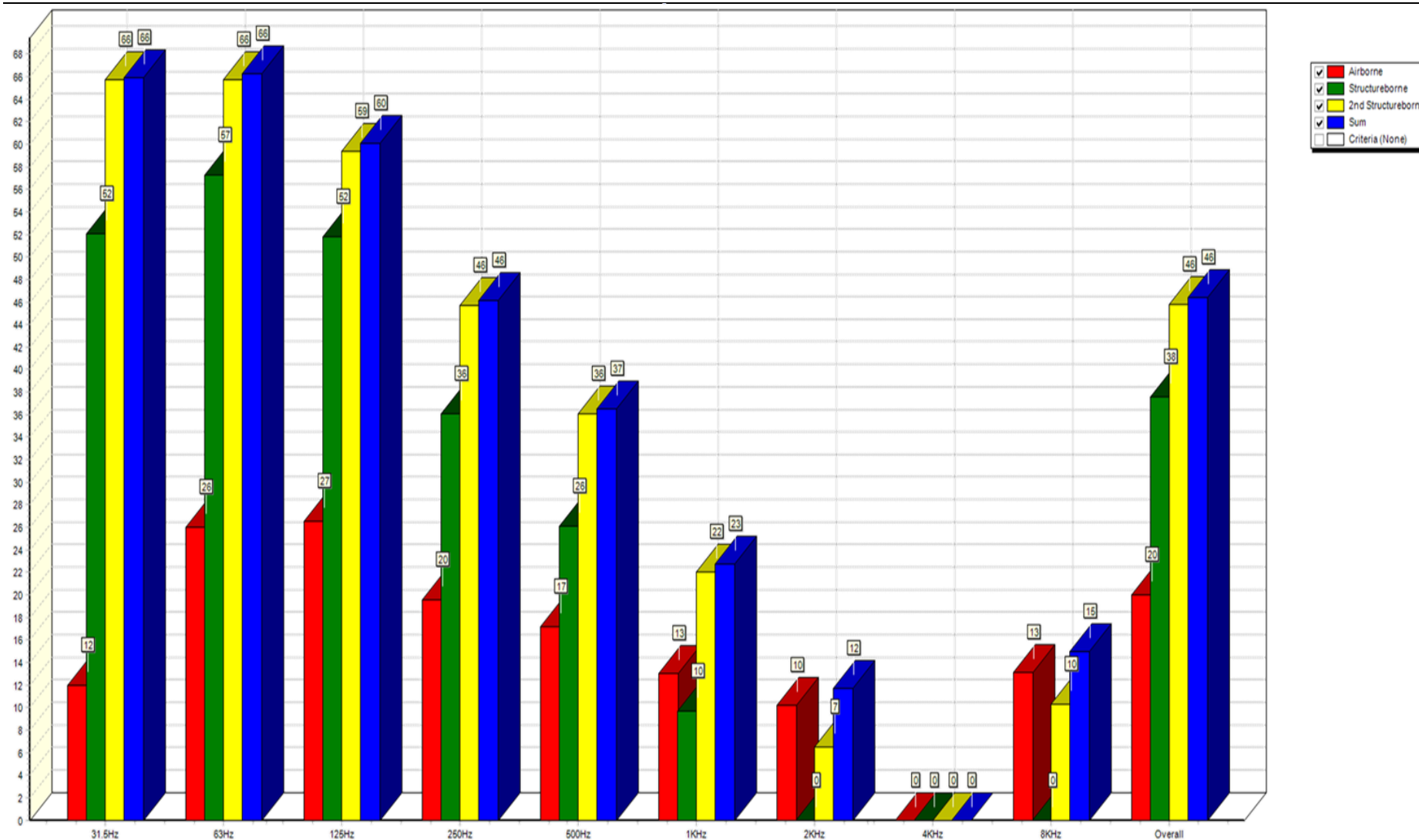
Slika 41. Razine buke za prostor kormilarnice (brod u luci, sa izolacijom)
