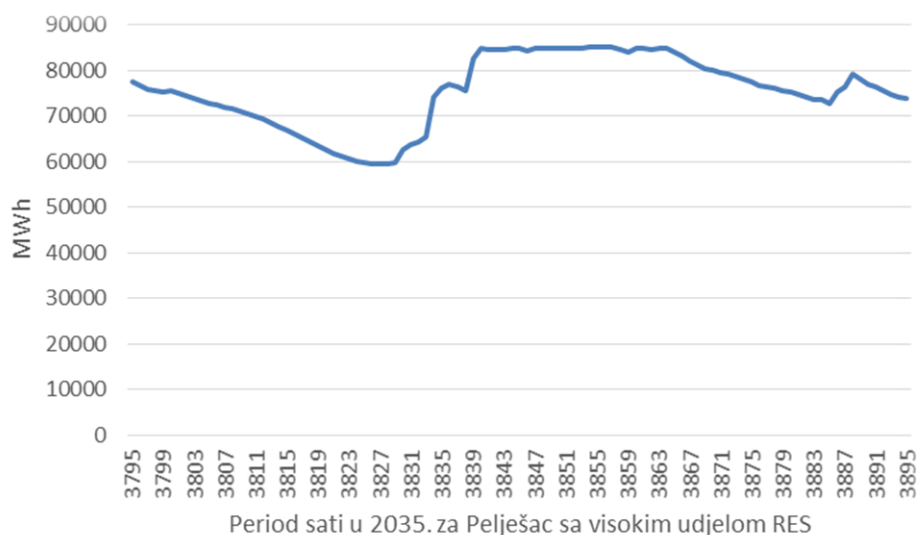
Slika 55 Kapaciteti baterija. Pelješac 2035. sa visokim udjelom OIE
