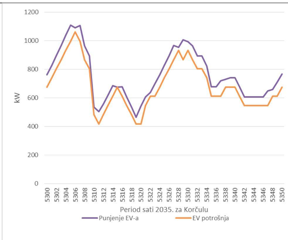
Slika 49 Period od 50 sati za Korčulu 2035. godine u umreženoj izvedbi, detaljan pogleda na ponašanje EV-a
