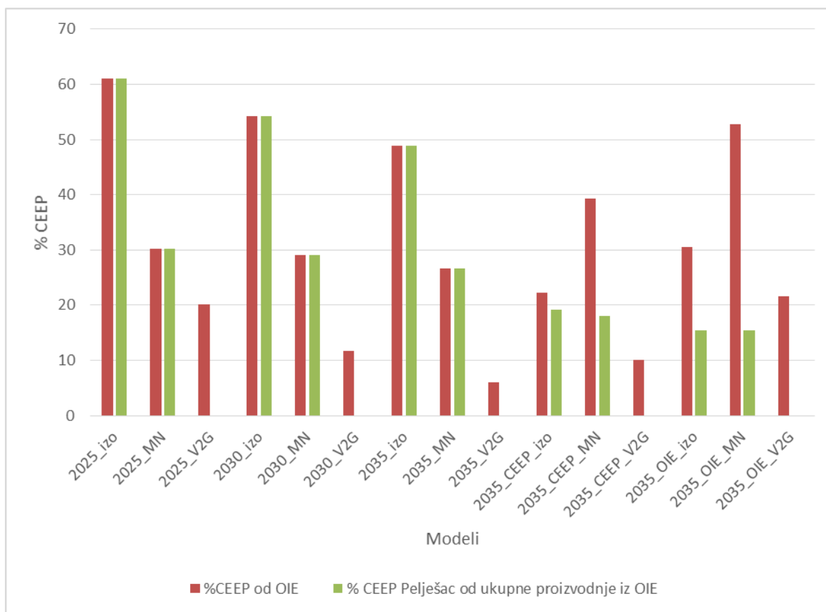
Slika 58 Analiza CEEP-a u svim modelima, izoliranim, dobivenim MultiNode umrežavanjem i umreženim sa V2G sustavom
