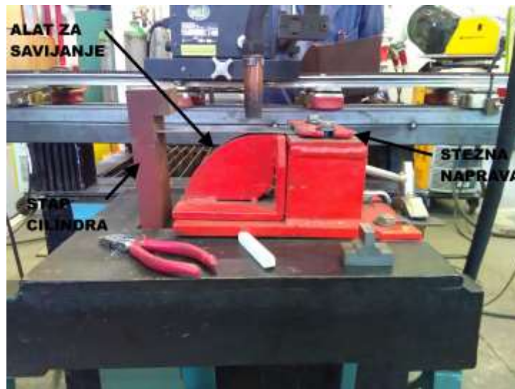
Slika 22. Uređaj za Varestraint
