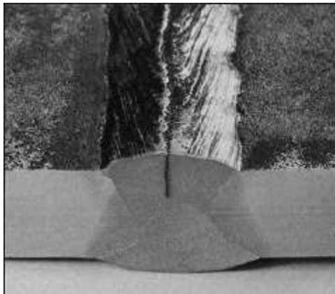
Slika 4. Vruća pukotina [8]
