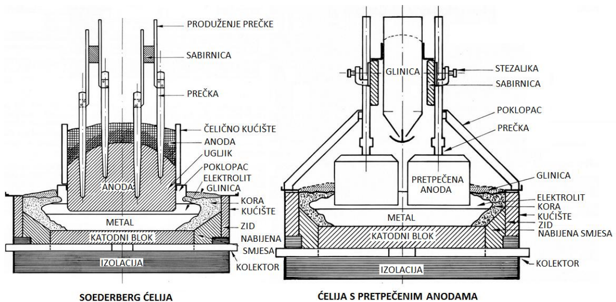
Slika 6. Ćelije za elektrolizu
