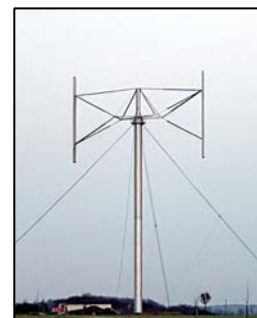
Slika 3.5. H-tip turbine
