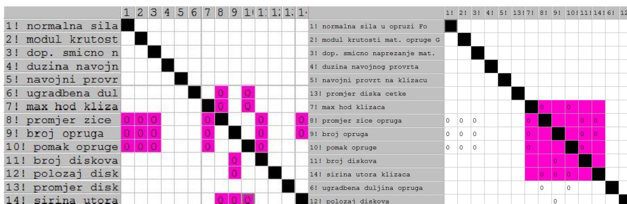
Slika 41: Particioniranje parametara mehanizma za poliranje prirubnice u alatu PSM 32 (lijevo prije partitioniranja, desno nakon partitioniranja)
