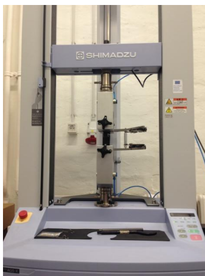
Slika 52. Kidalica za ispitivanje smične čvrstoće „Shimadzu“
