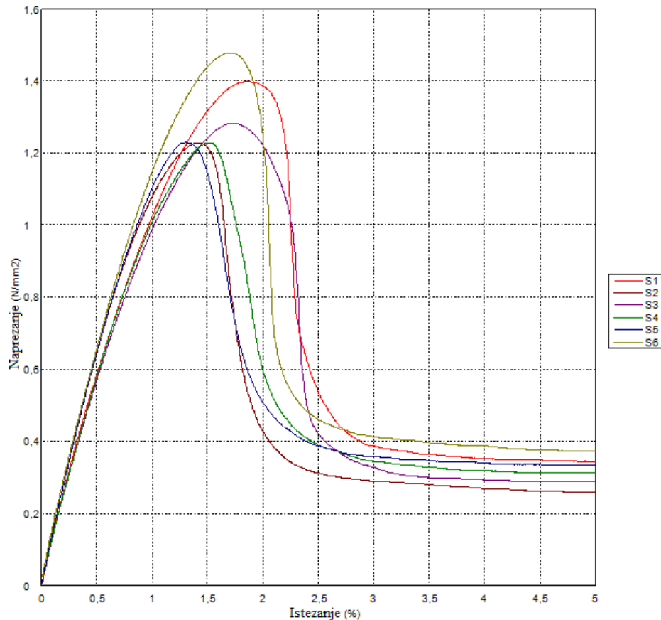
Slika 56. Dijagram naprezanje-istezanje
