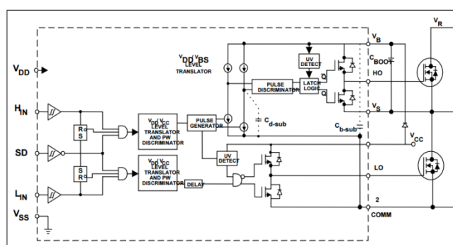
Slika 49. Shematski prikaz integriranog sklopa IR2110
