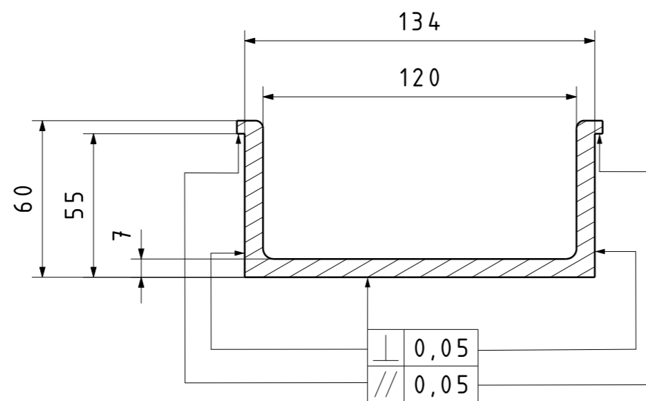
Presjek A-A
