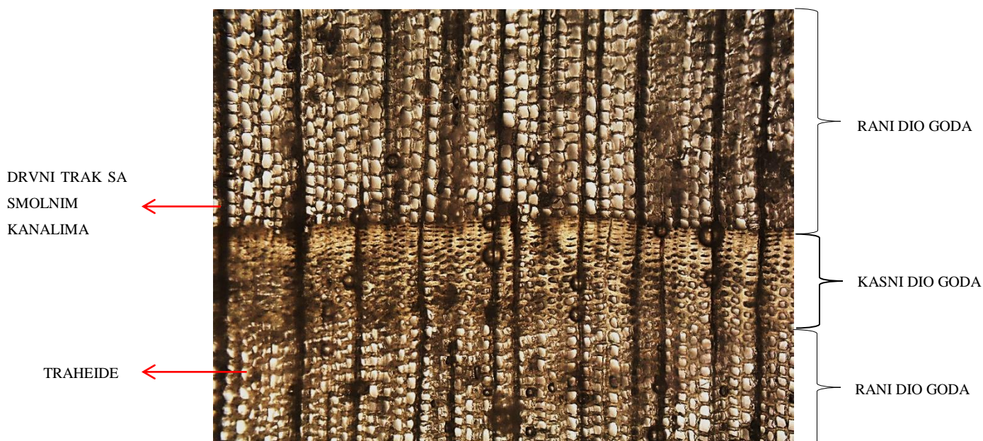
Slika 4.18. Mikrstruktura poprečnog presjeka ariša
