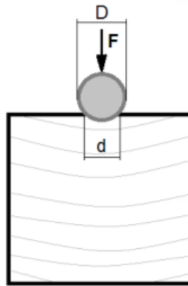
Slika 3.9. Shematski prikaz mjerenja tvrdoće po Brinellu [4]
