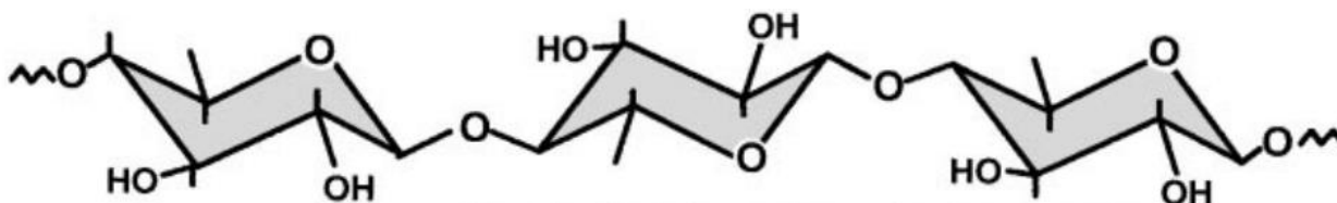
Slika 2.19. Hemiceluloza [5]
